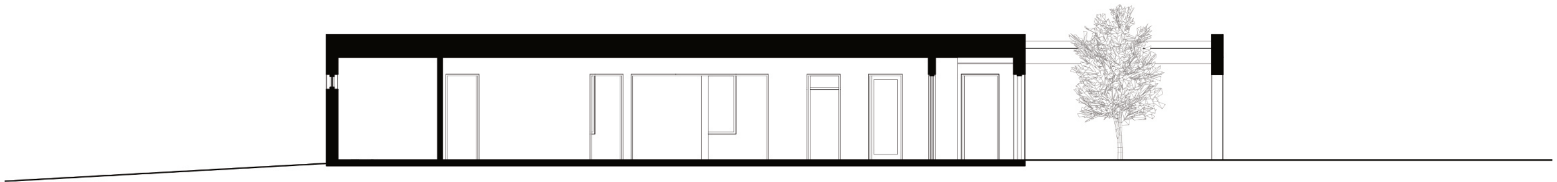
Snið D-D gegnum gang og aðkomugarð
