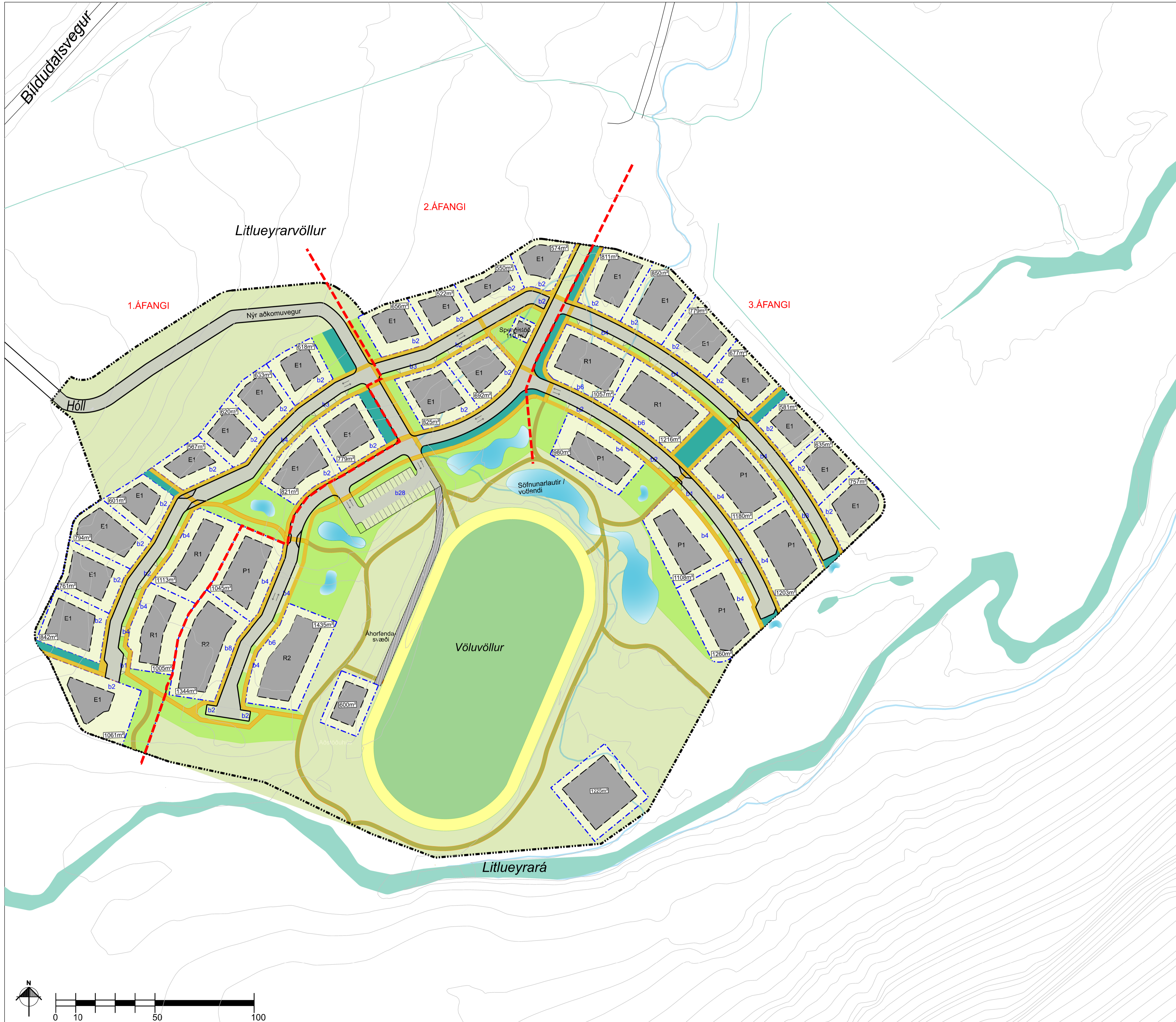
Deiliskipulagsuppdráttur Mkv 1:1000
